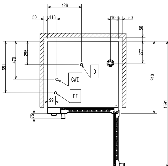
Boven aanzicht
